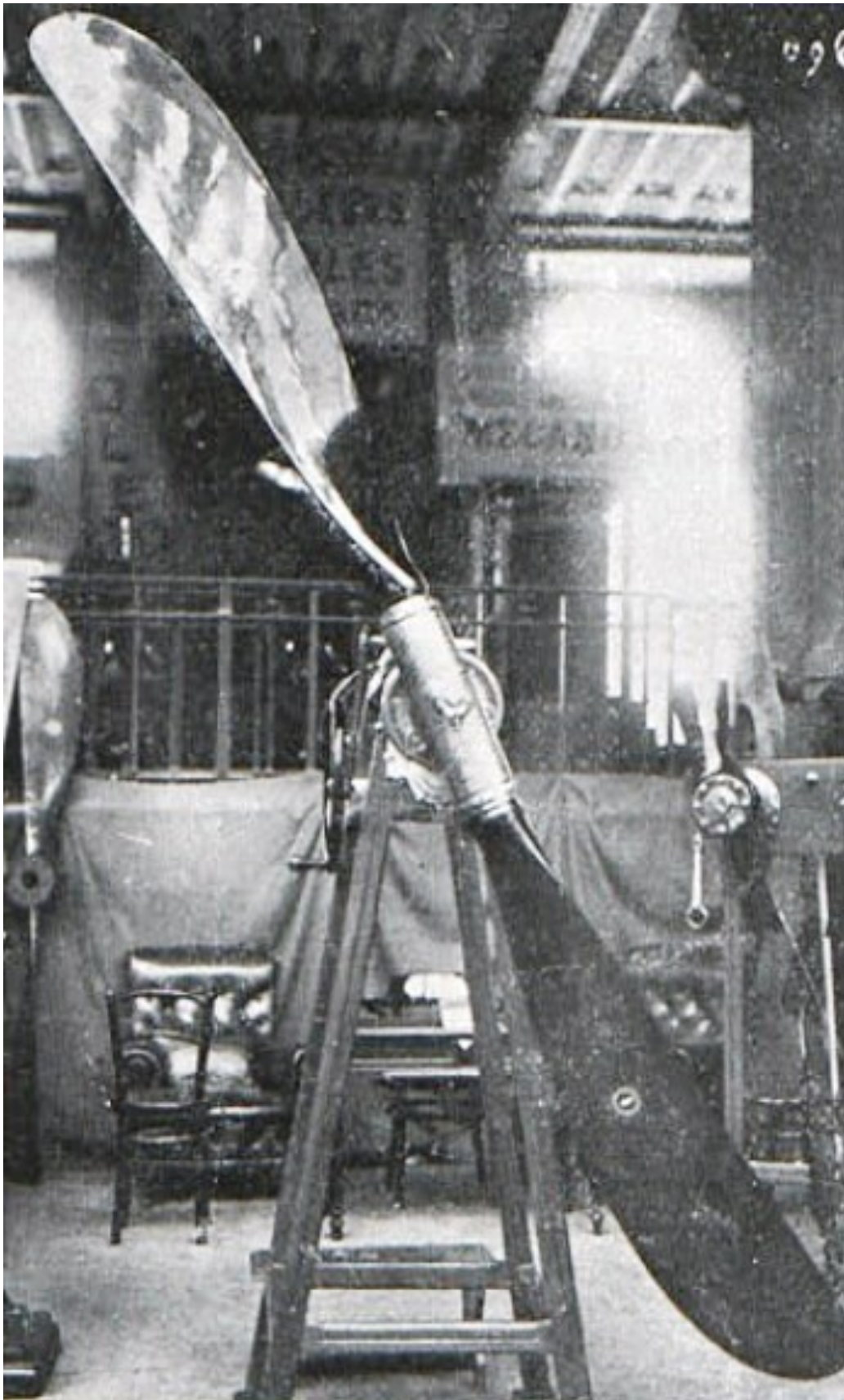
Hélice "governable" desde a bordo y en marcha 750
